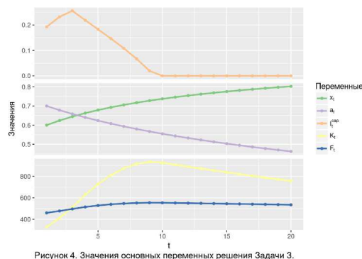
Рисунок 4. Значения основных переменных решения Задачи 3.
