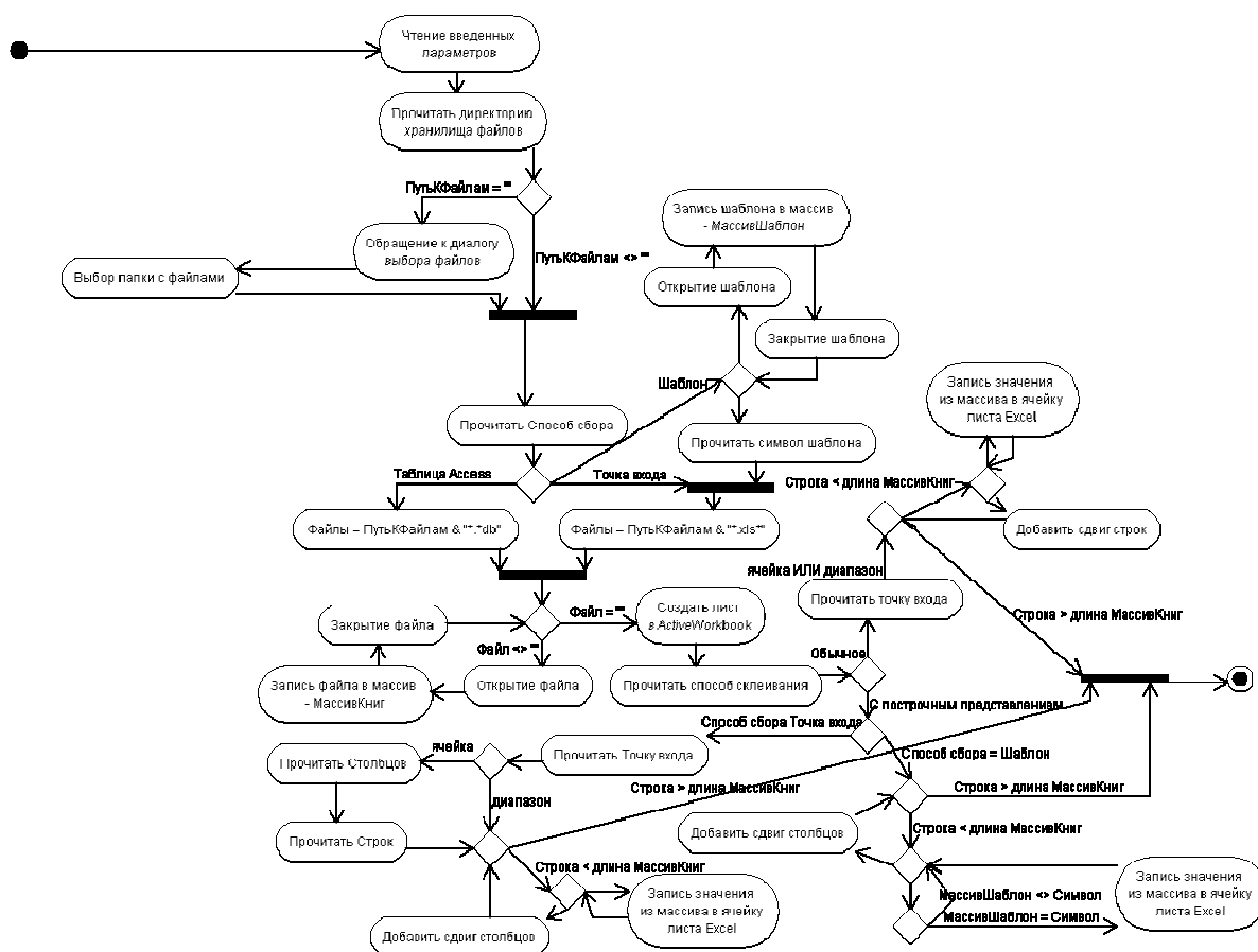
Рис. 4. Алгоритм работы команды «Собрать файл»
